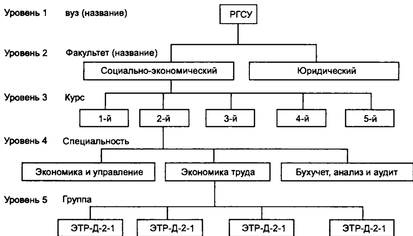
Рис. 2.4. Пример иерархической структуры данных
