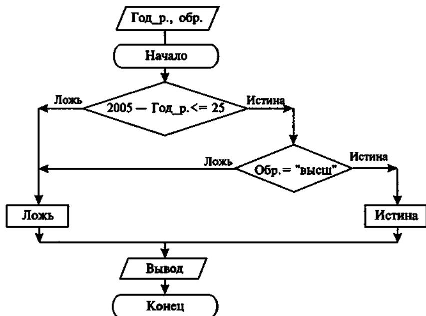
Рис. 6.20. Блок-схема алгоритма решения задачи отбора кандидатов (Пример 1)
