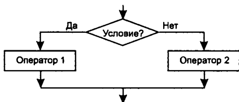
Рис. 2.11. Структура ветвления
