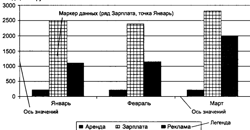
Рис. 6.42. Объекты диаграммы
